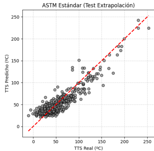
Figura 4.2: Ecuación de la norma ASTM E900-15 estandarizada.
