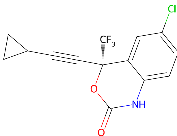
208 efavirenz
