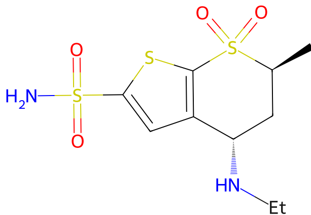
204 dorzolamide
