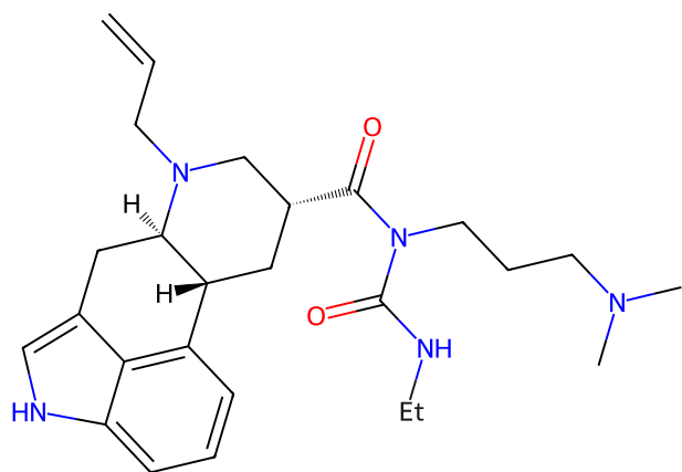
209 cabergoline
