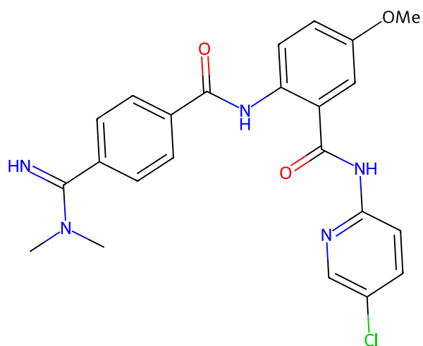
201 betrixaban
