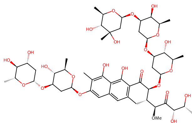
206 plicamycin
