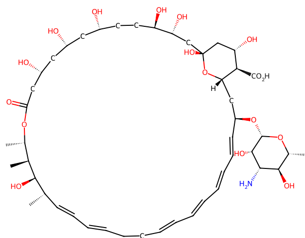
202 nystatin A1
