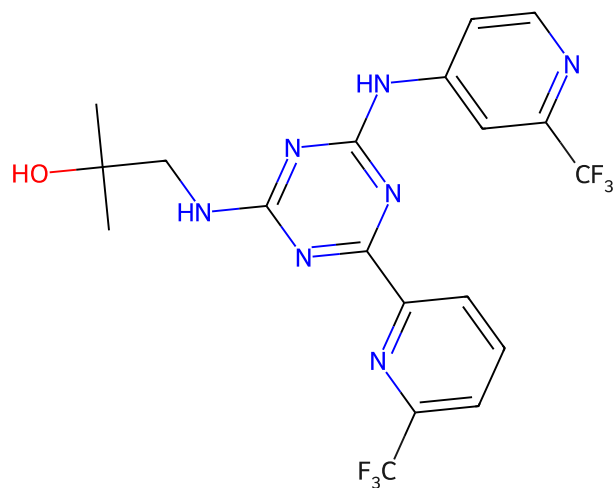
266 enasidenib
