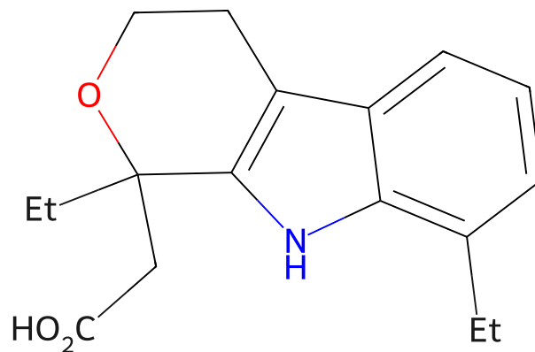
298 etodolac
