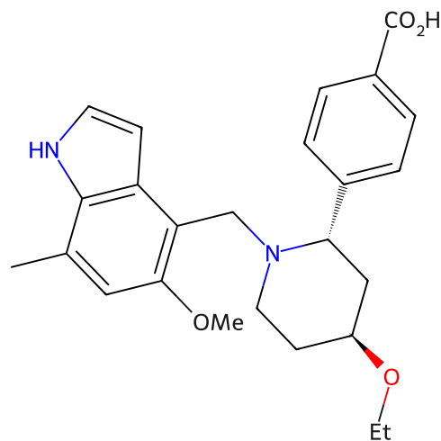
296 iptacopan
