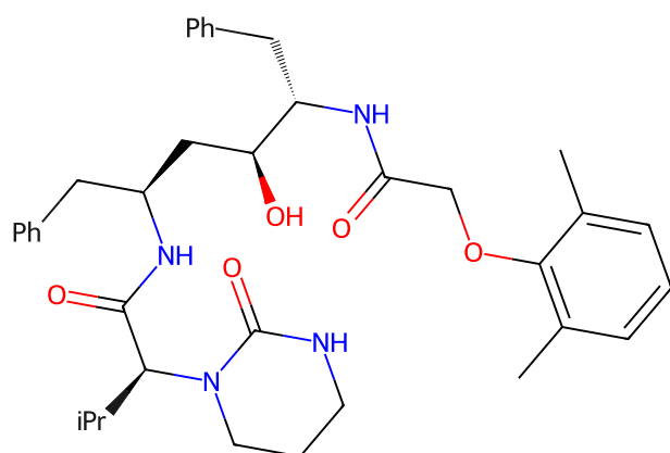
305 lopinavir
