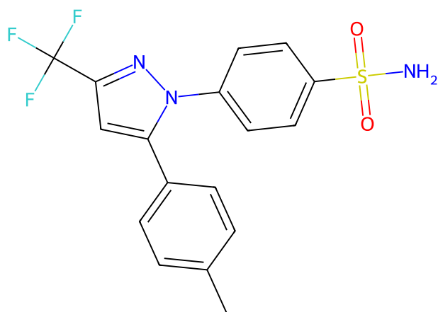
51 celecoxib
