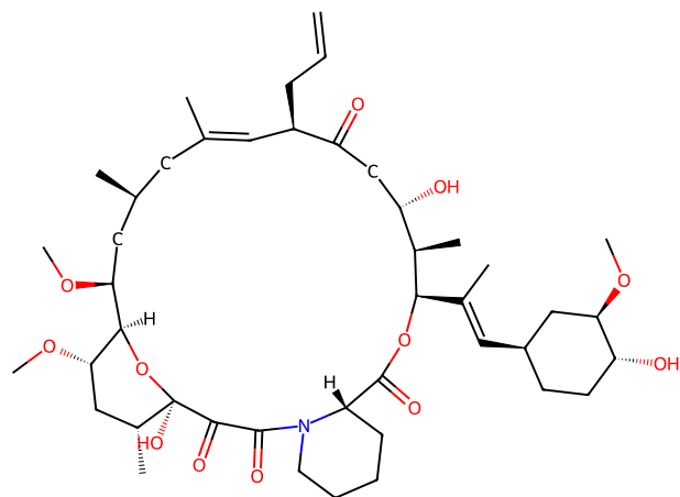
324 tacrolimus
