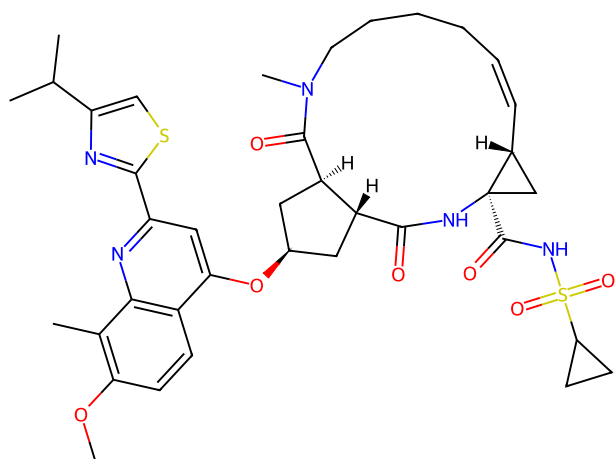
322 simeprevir
