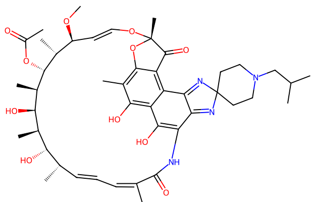
320 rifabutin
