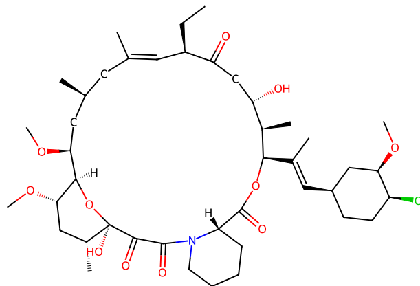
319 pimecrolimus
