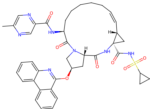
318 paritaprevir
