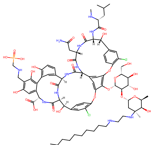
326 telavancin
