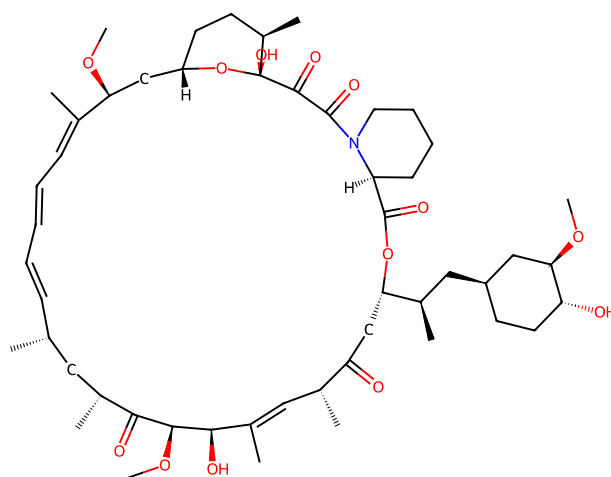
323 sirolimus
