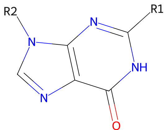
477 scaffold of ganciclovir
