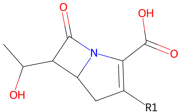
490 scaffold of imipenem
