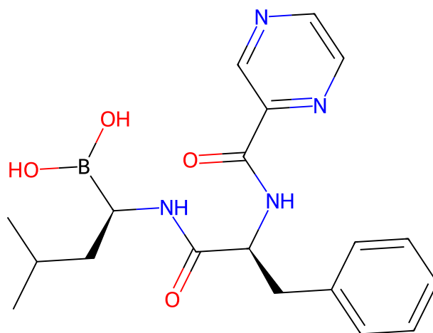
118 bortezomib
