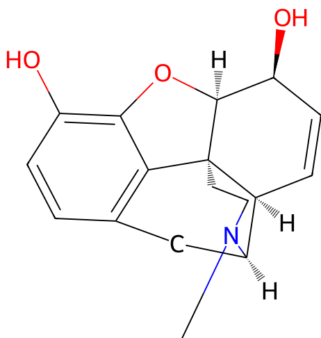
133 morphine
