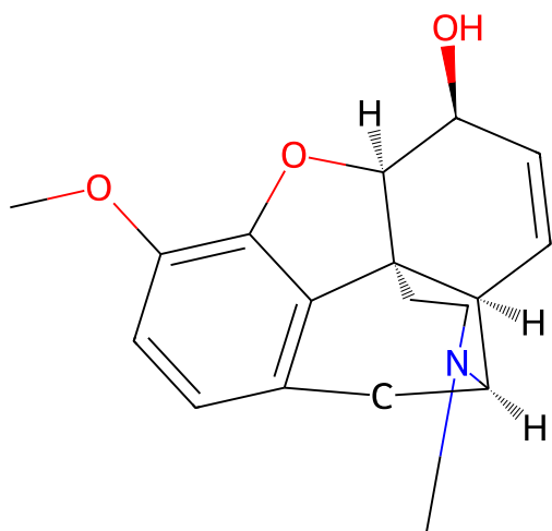
129 codeine
