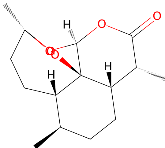
128 artemisinin
