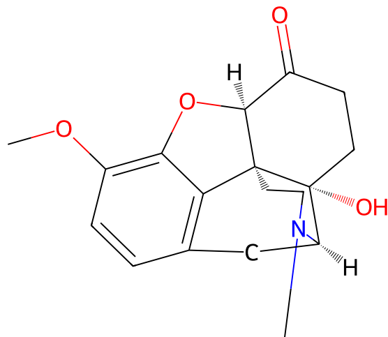
135 oxycodone
