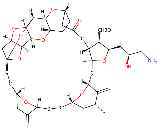
926 eribulin
