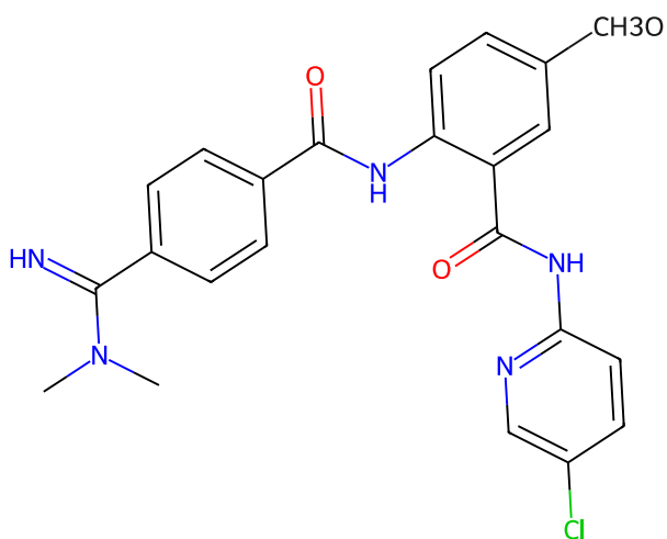
932 betrixaban
