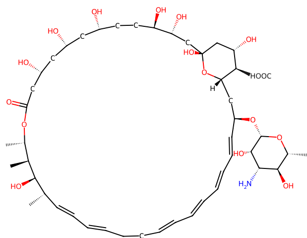
933 nystatin A1
