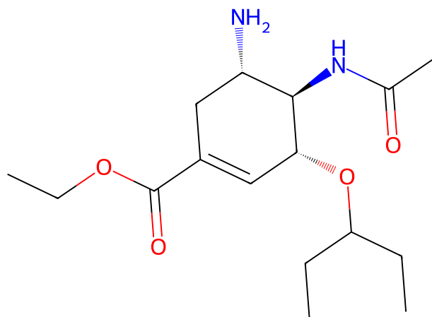
94 oseltamivir
