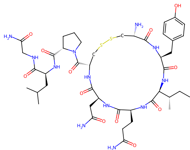
97 oxytocin
