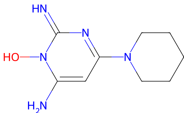
91 minoxidil
