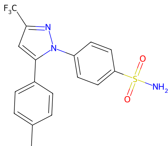
95 celecoxib
