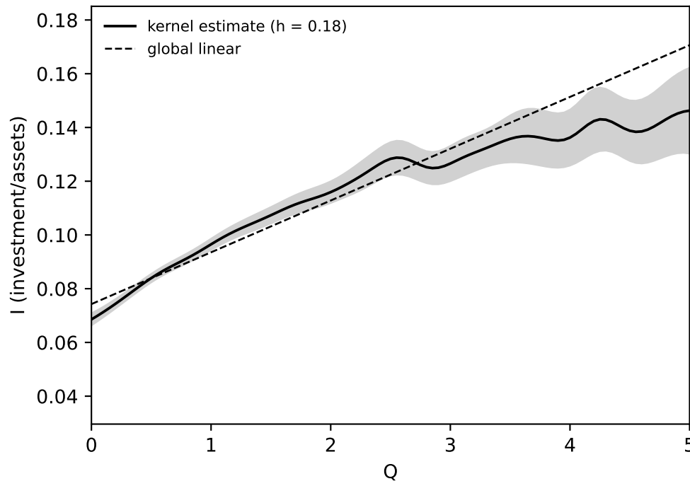
(a) Nadaraya-Watson
