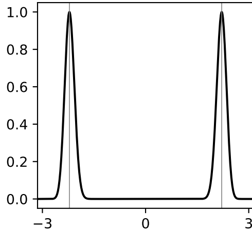
m=40, n=10
