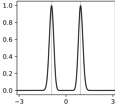
m=10, n=40
