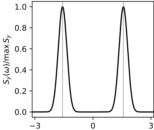
m=10, n=10
