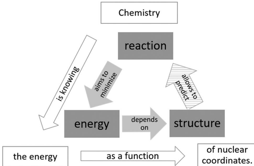
Abb. 2: Schema der chemischen Zusammenhänge zwischen chemischer Reaktion, Energie und Struktur basierend auf Goodwin (2007) und Jensen (2007)
