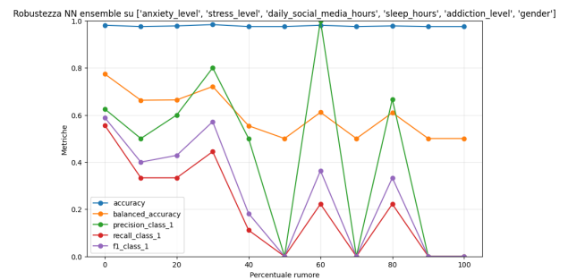
(b) Neural Network, feature migliori
