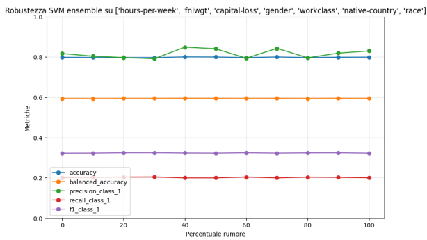
(a) SVM, feature peggiori
