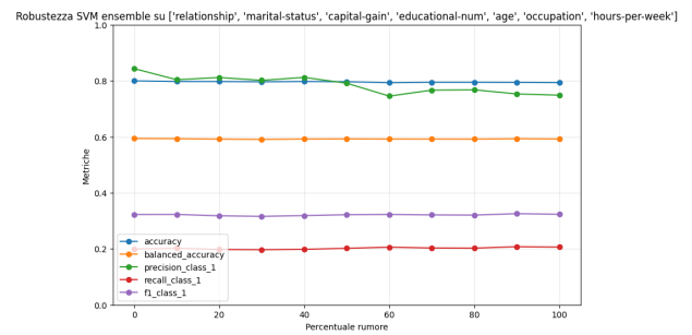
(b) SVM, feature migliori
