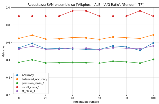
(a) SVM, feature peggiori
