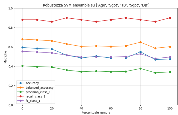
(b) SVM, feature migliori
