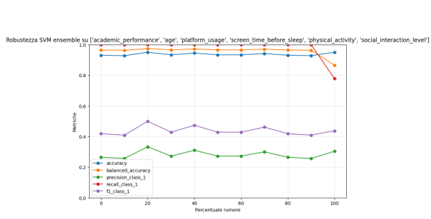
(a) SVM, feature peggiori
