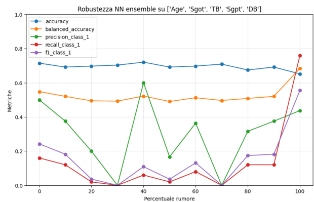
(b) Neural Network, feature migliori
