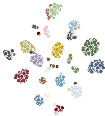
Ovenbird (ours)
