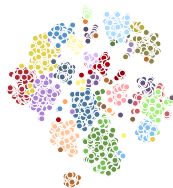
Perch V2
