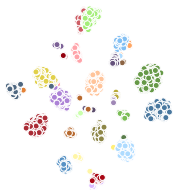
Ovenbird (ours)
