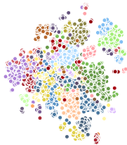
BirdNET
