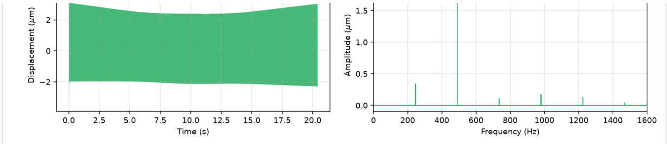
الشكل 15 — الحالة S: (4900 tr/min, a_p = 0.30 mm) بلا تحكّم تتباعد عند 0.085 s برجفان عند 534 Hz: FOPID يُثبت الممرّ كلّهُ 6.6) بطيف لا يحوي سوى توافقيات مرور الأسنان؛ وADRC-FOPID يتباعد عند 0.114 s.
