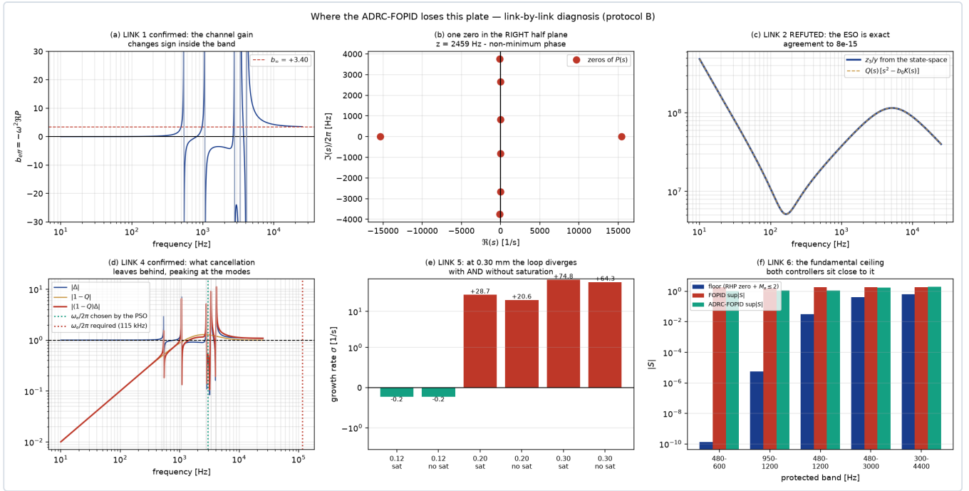
الشكل 25 — التشخيص حلقة حلقة: (a) الكسب الفعّال يقلب إشارته، (b) صفر في النصف الأيمن، (c) ال ESO مضبوط تمامًا، (d) المتبقي غير المُغلى يبلغ ذُراه عند الرنينات، (e) التثبيط عَرَض، (f) السقف الأساسي.
