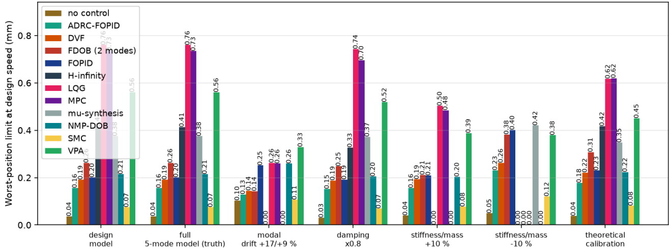
الشكل 32 — المتانة عبر سبع حالات اضطراب. الأعمدة الصفيرة انهيار تام لا حد صغير.
