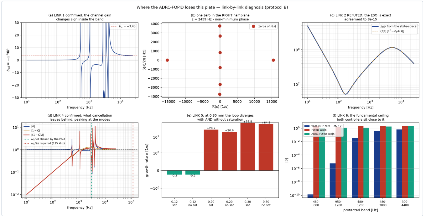
الشكل 25 — التشخيص حلقةً حلقة: (a) الكسب الفعّال يقلب إشارته، (b) صفر في النصف الأيمن، (c) ال ESO مضبوط تمامًا، (d) المتبقي غير المُلغى يبلغ ذُراه عند الرنينات، (e) التشيع عَرَض، (f) السقف الأساسي.
