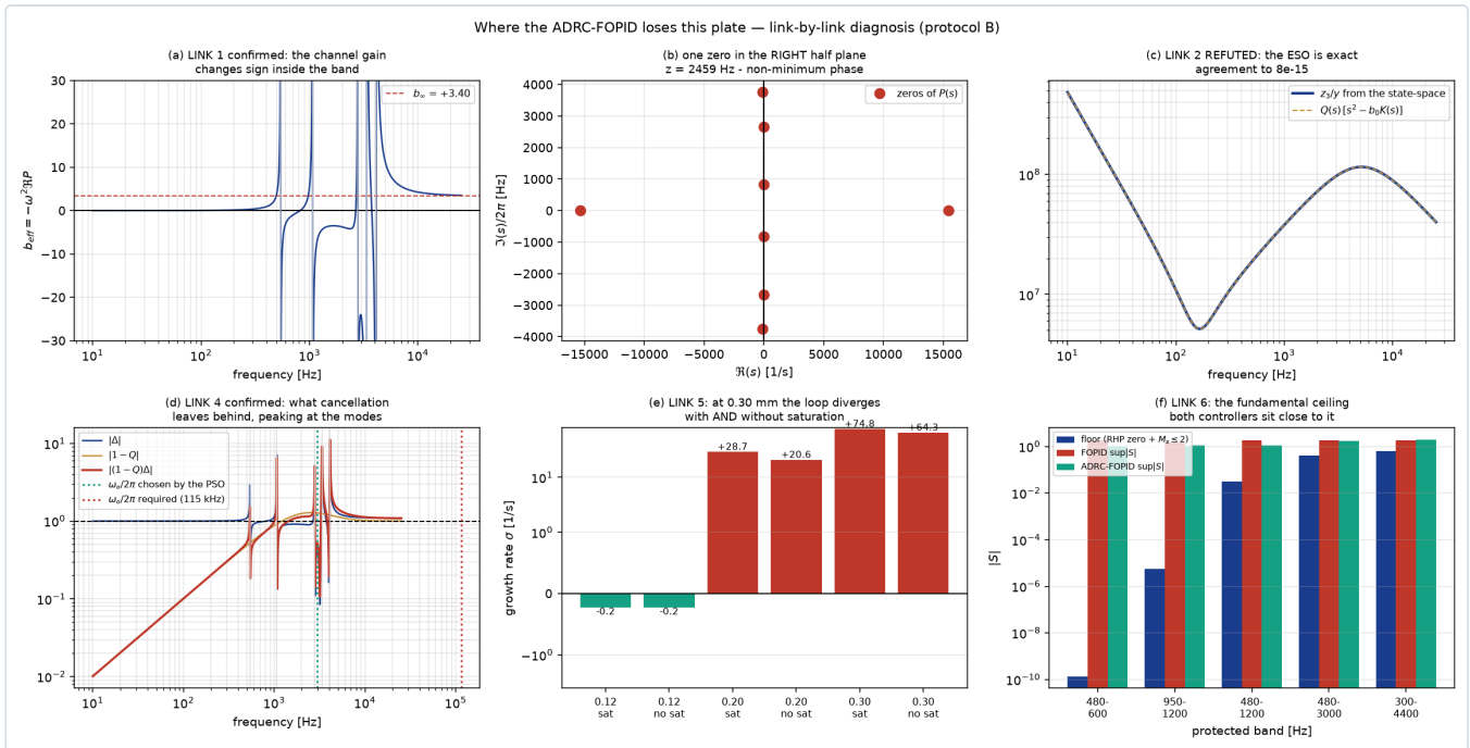
الشكل 25 — التشخيص حلقةً حلقة: (a) الكسب الفعّال يقلب إشارته، (b) صفر في النصف الأيمن، (c) ال ESO مضبوط تمامًا، (d) المتبقي غير المُلغى يبلغ ذُراه عند الرنينات، (e) التثنيع عَرَض، (f) السقف الأساسي.
