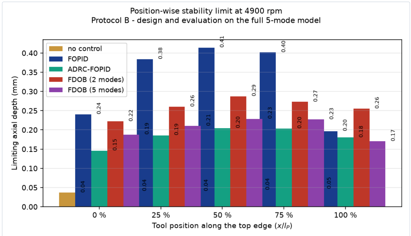
الشكل 30 — ملص الموضع: FOPID مُدَبَّب، والمُلاحَظ المودالي مُسطّح — وهذا يقرّر أيّ مقياس يفوز به كلّ منهما.
