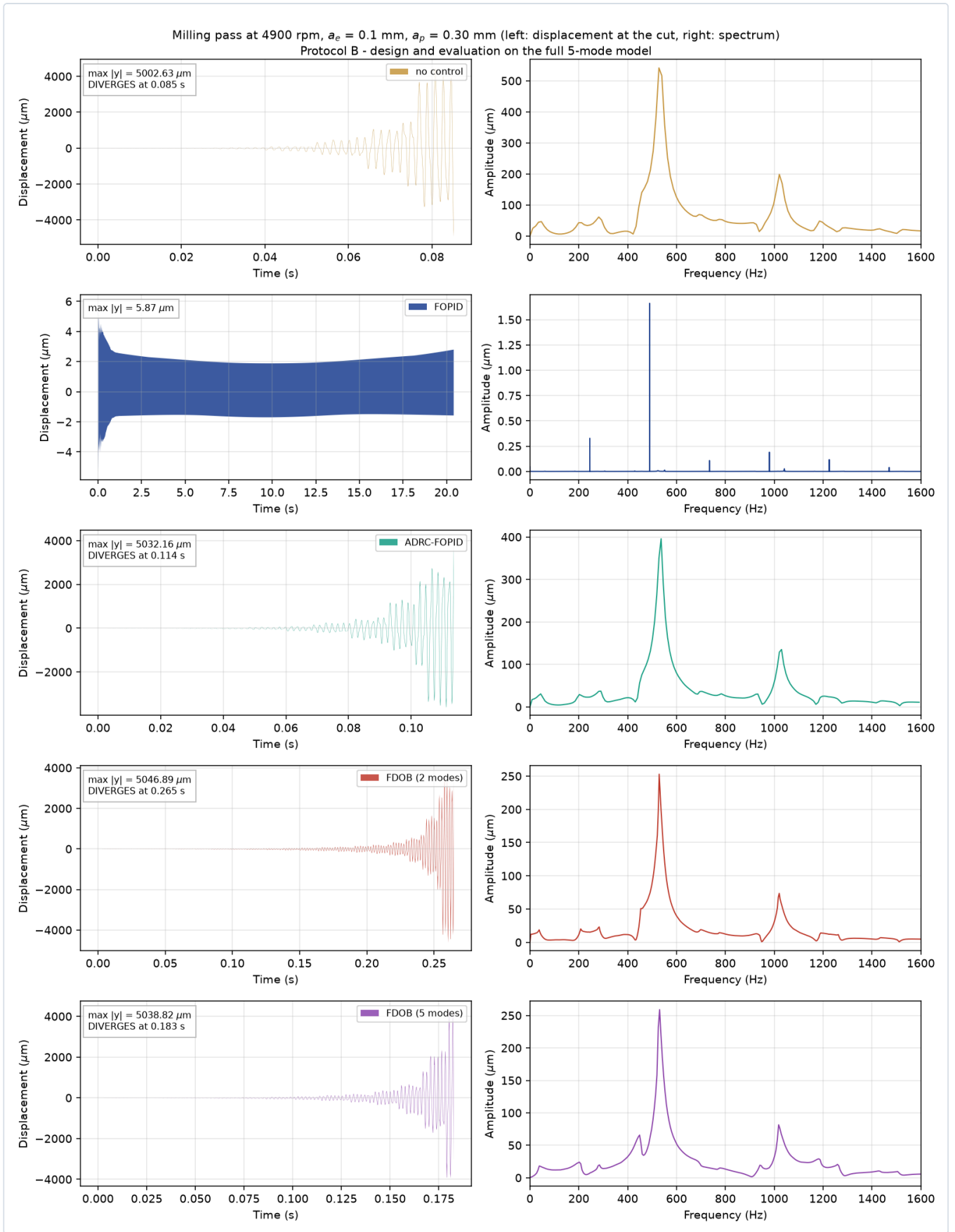
الشكل 15 — الحالة (4900 tr/min, a_p = 0.30 mm) S: بلا تحكم تتباعد عند 0.085 s برجفان عند 534 Hz؛ FOPID يُبَيِّت الممرَّ كَـ 6.6) بطيف لا يحوي سوى توافقيات مرور الأسنان؛ وADRC-FOPID يتباعد عند 0.114 s.
