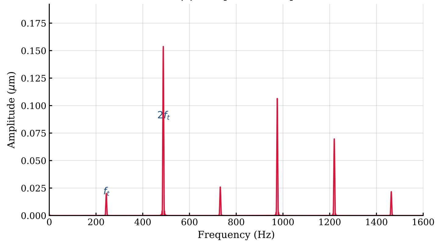
(d) FFT[DARC-MPC]
