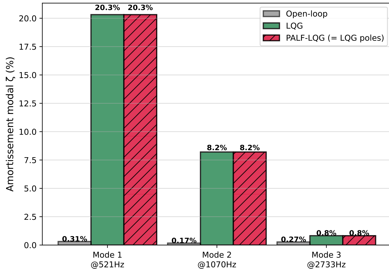
Amortissement modal en boucle fermée (S1)
