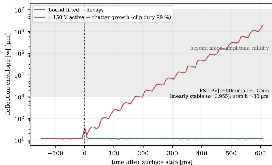
(d) saturation island: causal demonstration
