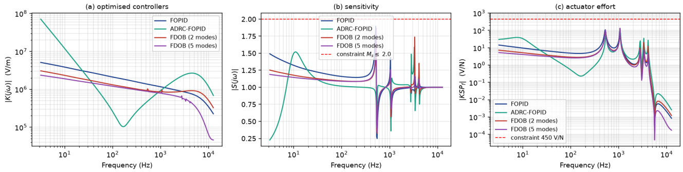
الشكل 21 — التوقيعات الترددية تحت القيود نفسها: |K| و |S| والجهد لكل نيوتن.
