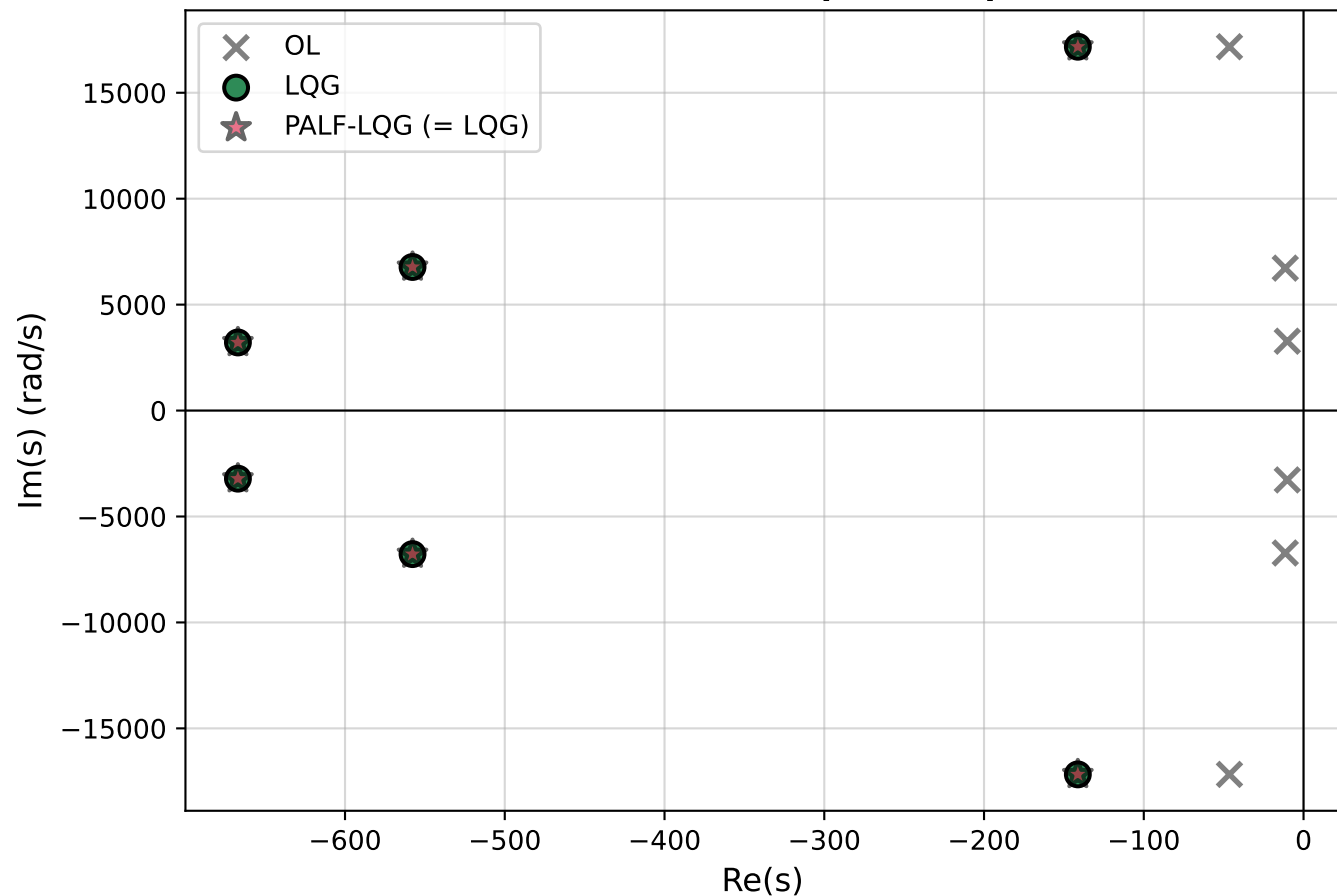
Pôles boucle fermée (plan complexe)
