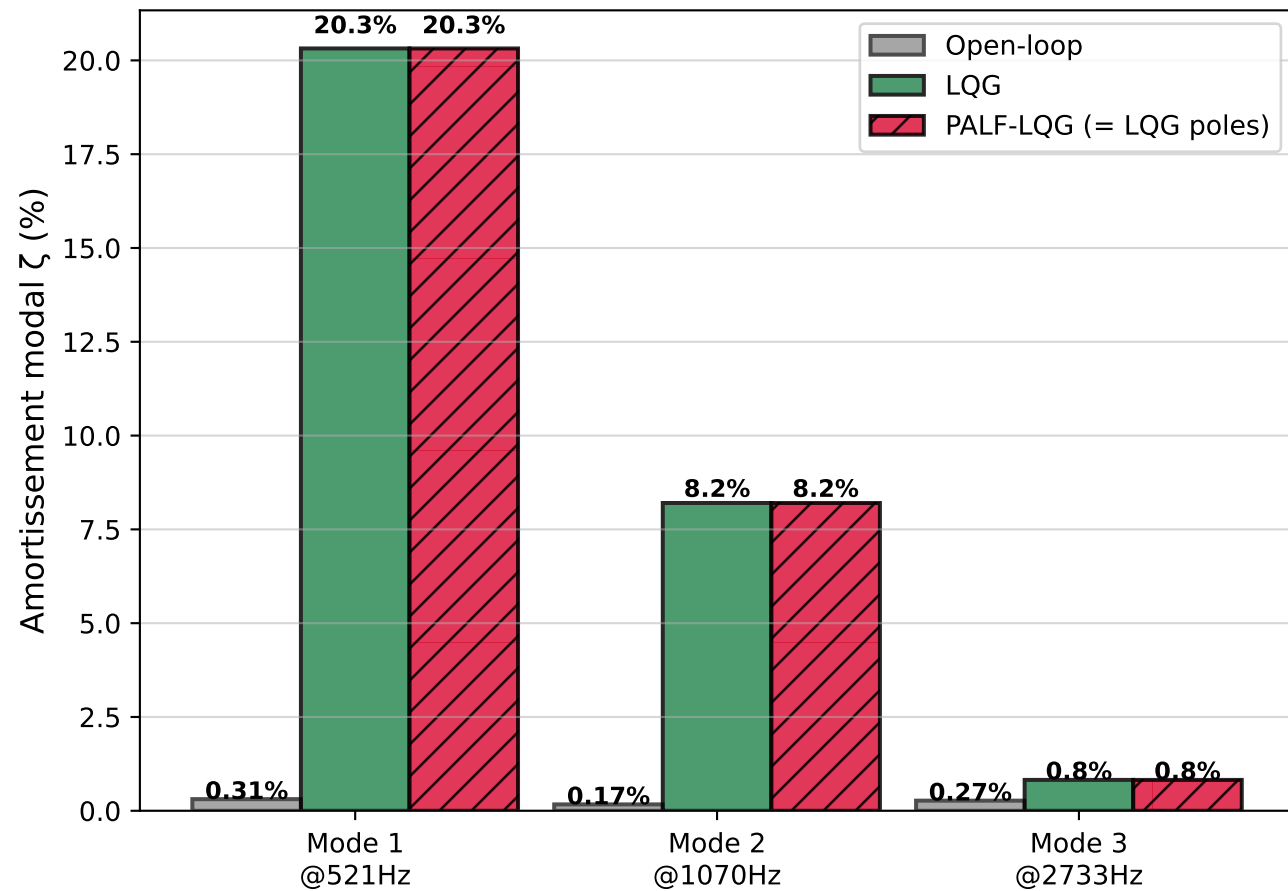
Amortissement modal en boucle fermée (S1)
