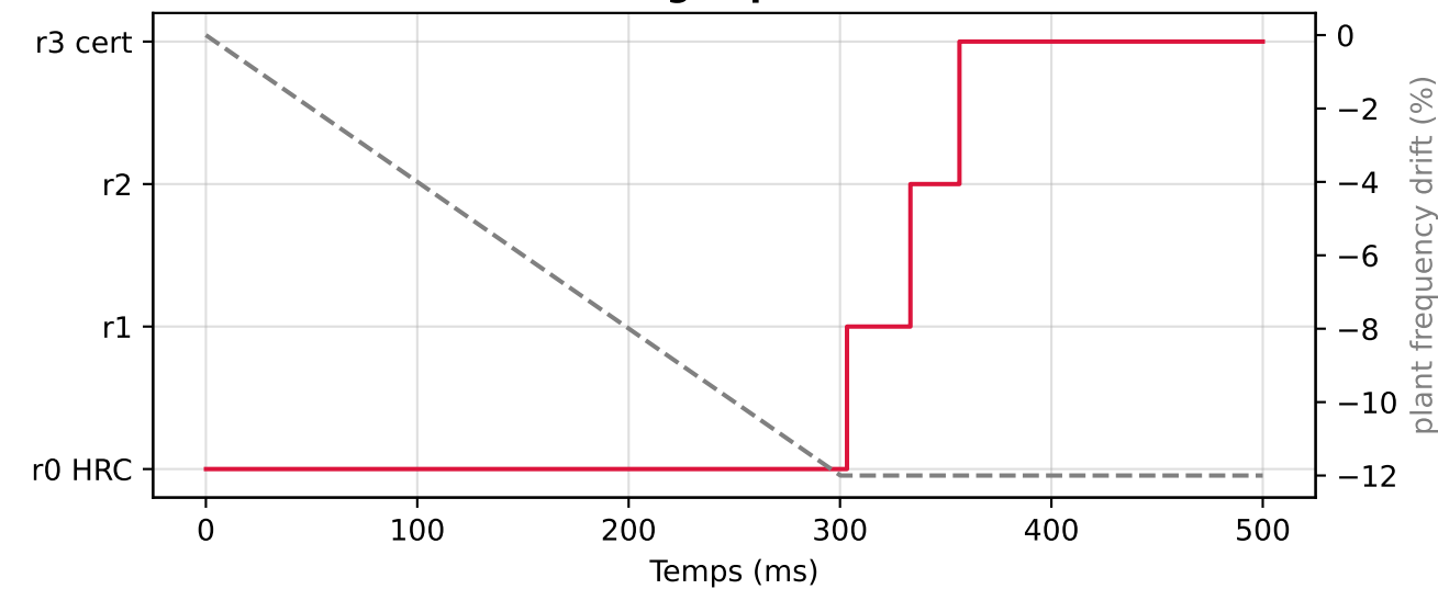
A-ESO-ADRC rung supervision under D2
