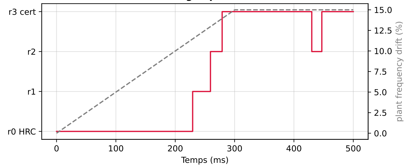
A-ESO-ADRC rung supervision under D1
