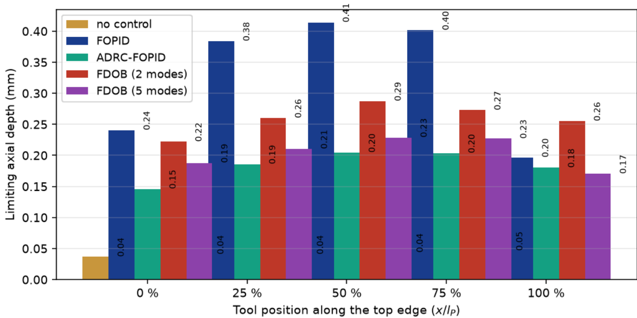
الشكل 29 — ملحق الموضوع: FOPID مُدَبَّب، والمُلاحَظ المودالي مُسطَّح — وهذا يقرَّر أيَّ مقياس يفوز به كلُّ منهما.
