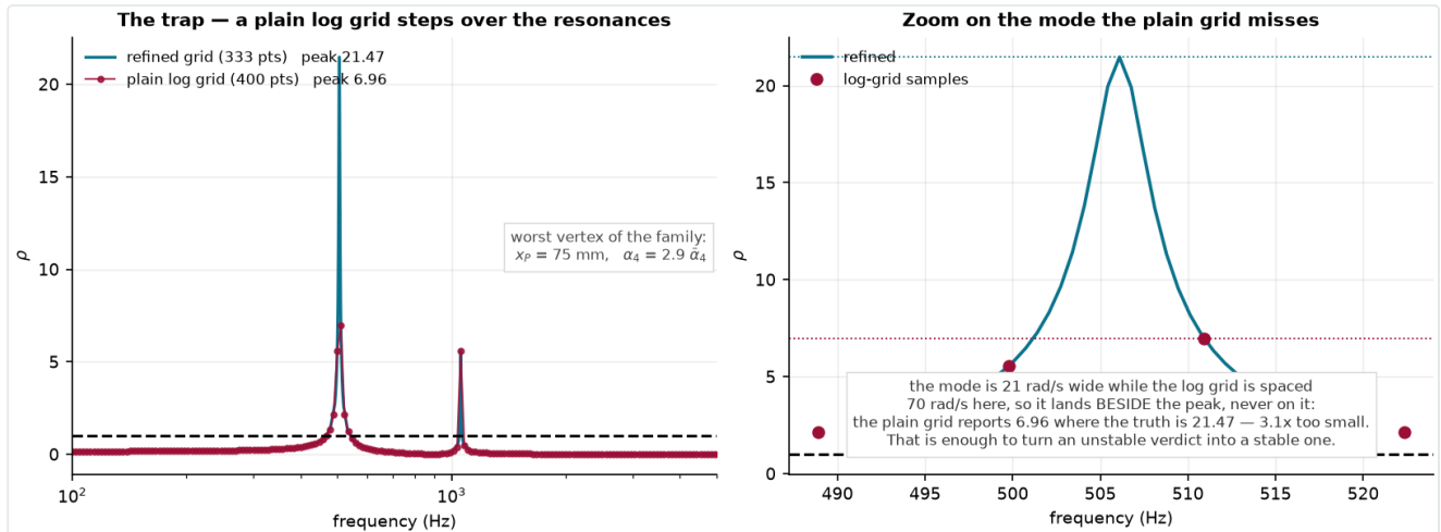
الشكل k2. الفخّ: شبكة لوغاريتمية بـ 400 نقطة تففز فوق الرنين عند أسوأ رأس فتُبَلِّغ 6.96 حيث الحقيقة 21.47. وفي التكبير موقع العينات – بجانب الذروة لا عليها.
