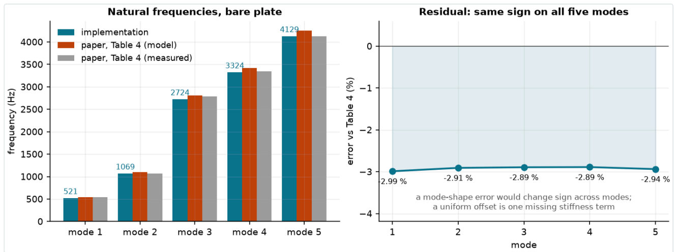
الشكل v1. التواترات الذاتية الخمس مقابل الجدول 4 في [1]، والبواقي إلى جانبها. الخطأ منتظم الإشارة على الأنماط الخمسة – وهذا توقيع حدّ صلابة عامّ مفقود، لا خطأ في أشكال الأنماط، إذ كان خطأ الأشكال سيقبّل إشارته بين نمط وآخر.
