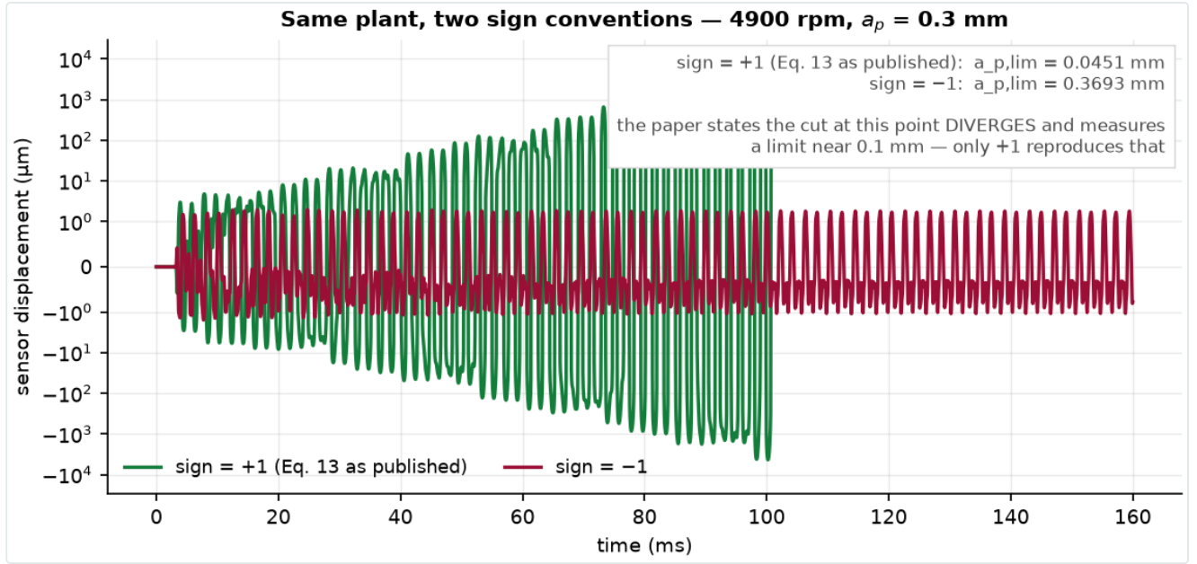
الشكل v5. المنظومة نفسها باصطلاحي الإشارة عند نقطة التشغيل: +1 يتباعد في 0.107 s، و-1 لا يتباعد إطلاقاً. والمرجع يقول إنَّ القطع هنا يتباعد ويقبس حدًّا قرب 0.1 mm — فالاصطلاح +1 وحده يعيد إنتاج ذلك.
