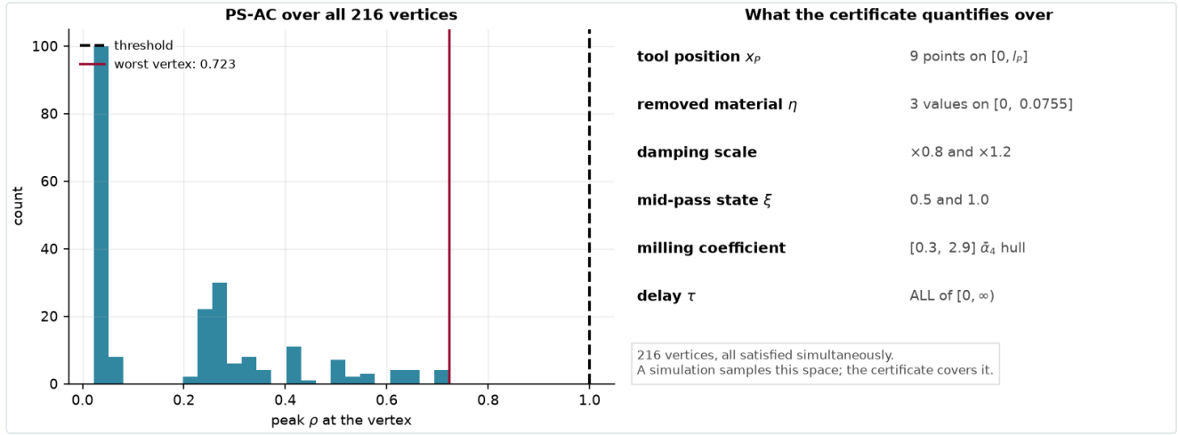
الشكل k5. توزيع الذروة على الرؤوس الـ 216 PS-AC، وما تُكَمِّمُه الشهادة إلى جانبه: الموضع، وإزالة المادة، والتخميد، وحالة منتصف الممر، وغلاف معامل القطع – وكل التأخيرات في آنٍ واحد.
