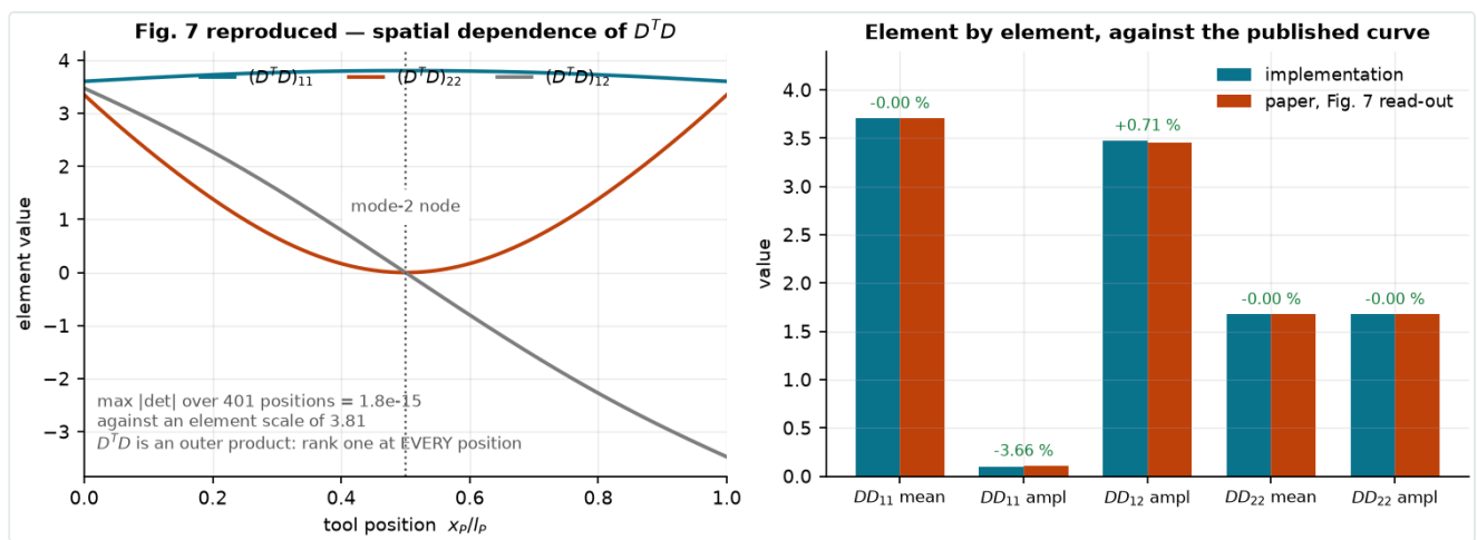
الشكل v3. الشكل 7 من [1] مُعادًا إنتاجه: عناصر D^T D على طول الحافة العليا. النمط الثاني يمرّ بعقدة عند المنتصف، فيسقط الحدّ التجديدي هناك؛ والمصفوفة رتبته واحد عند كل موضع ( |\det| \leq 1.8 \times 10^{-15} ) مقابل مقياس عنصر (3.81). واللوحة الثانية تقارن كل عنصر بقراءة الشكل المنشور.
