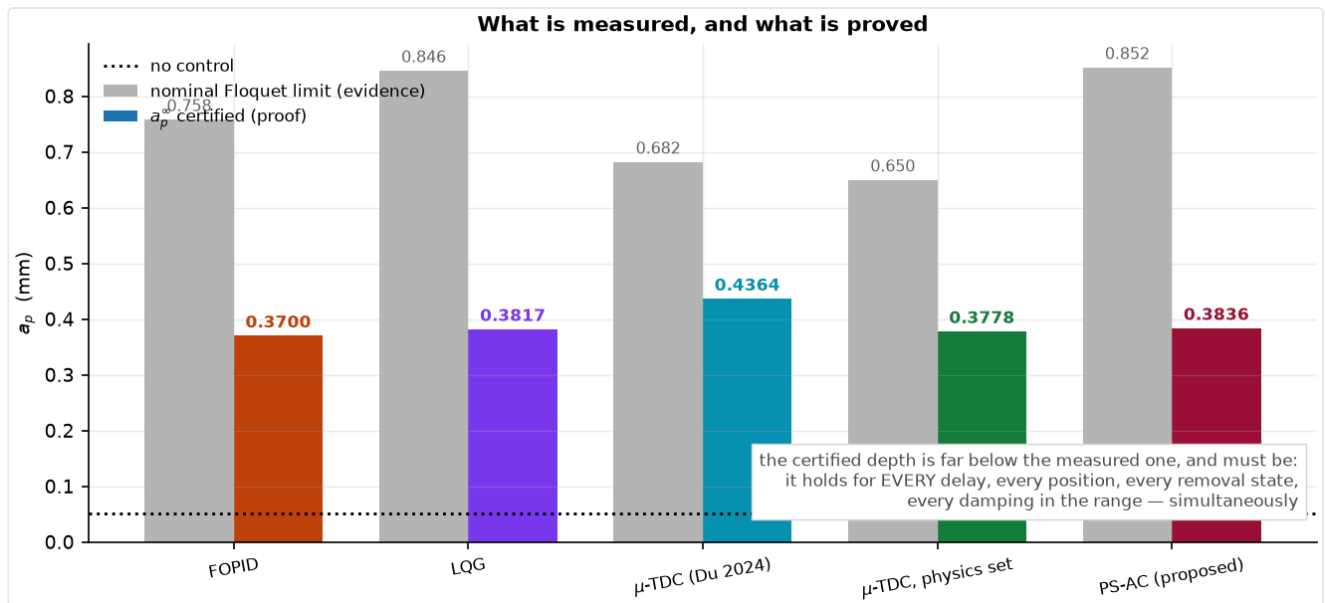
الشكل k3. ما يُقاس وما يُبرهن: حدّ فلوكيه الاسمي (رمادي) إلى جانب العمق المُصادق a_p^\infty (ملوّن). المُصادق أدنى بكثير ويجب أن يكون كذلك — فهو يصمد لكل تأخير وكل موضع وكل حالة إزالة وكل تخميد في آنٍ واحد.
