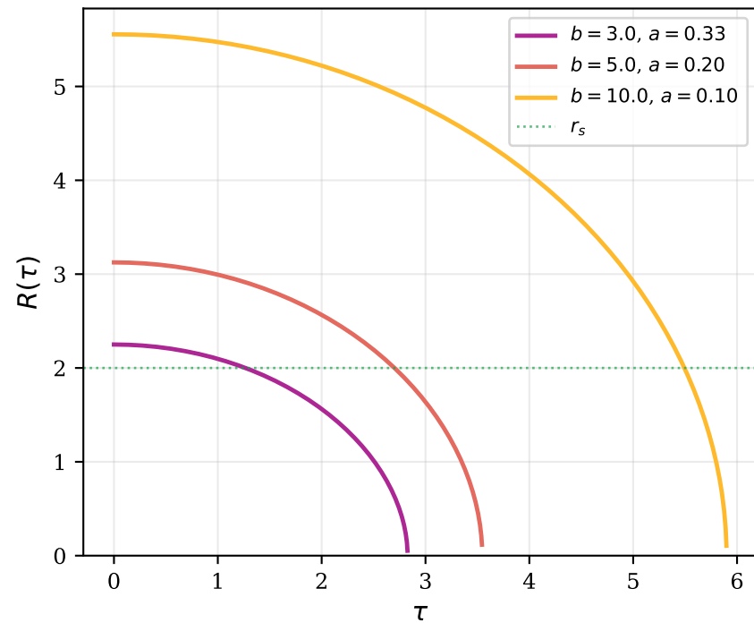
Trayectorias R(\tau)
