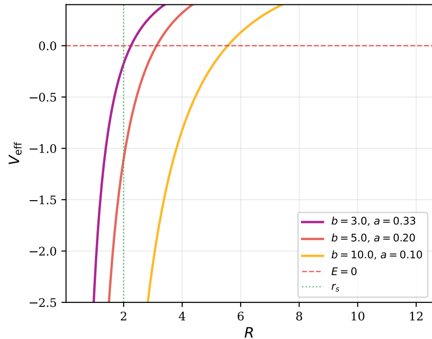
Potencial efectivo
