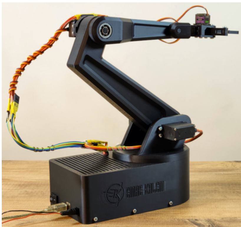
Obr. 2: Konštrukcia celého robotického ramena
