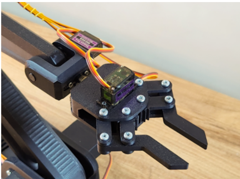
Obr. 3: Konštrukcia Gripera
