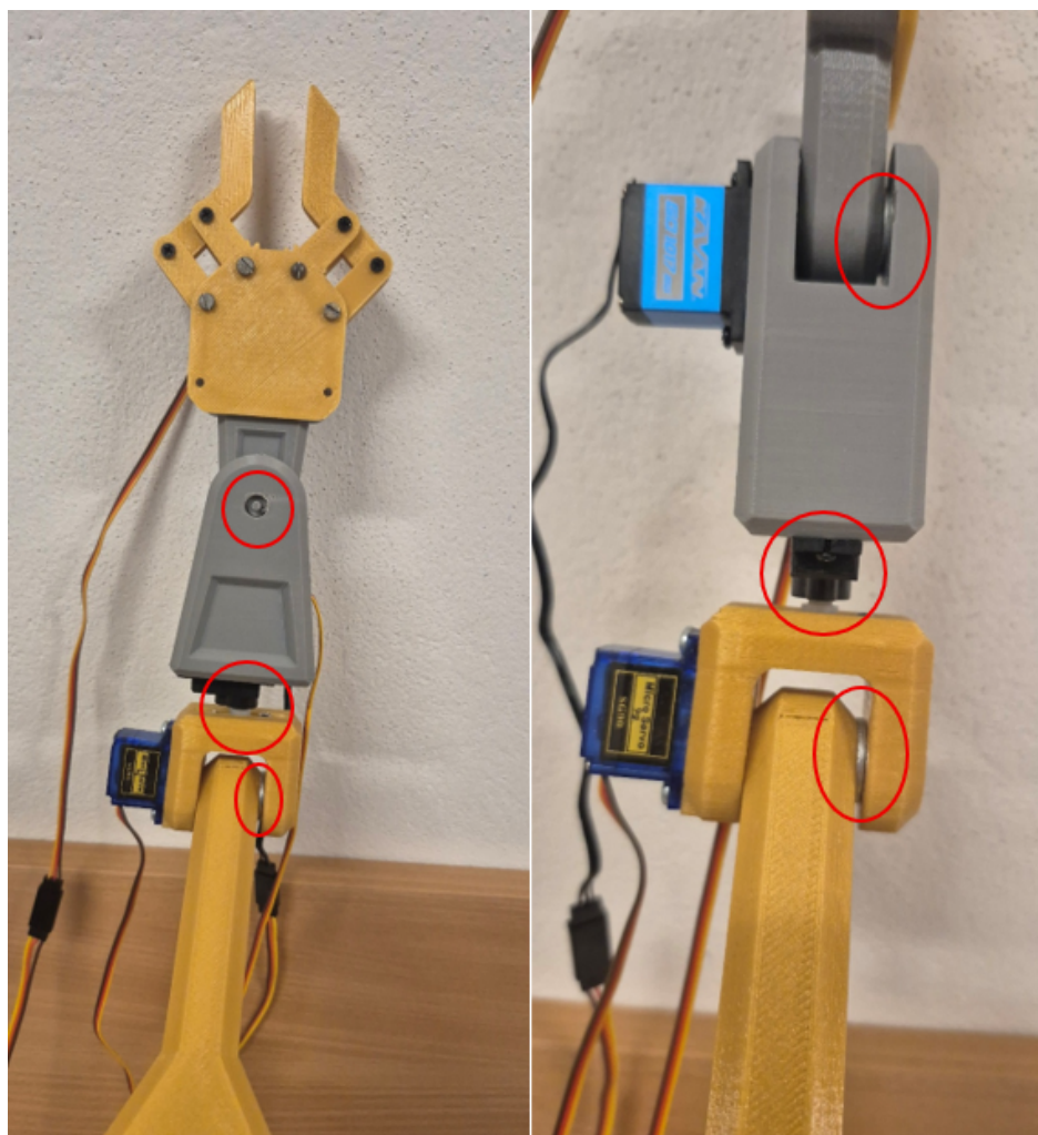
Obr. 7: Konštrukčné problémy ramena
