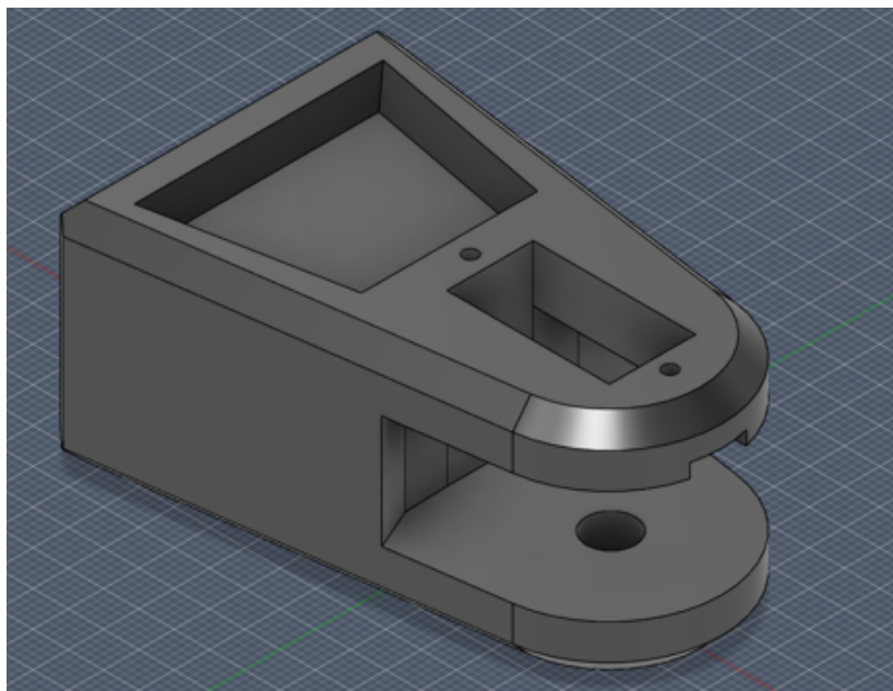
Obr. 4: Kľb na držanie mikroservo motorov pre osi "zä "y"
