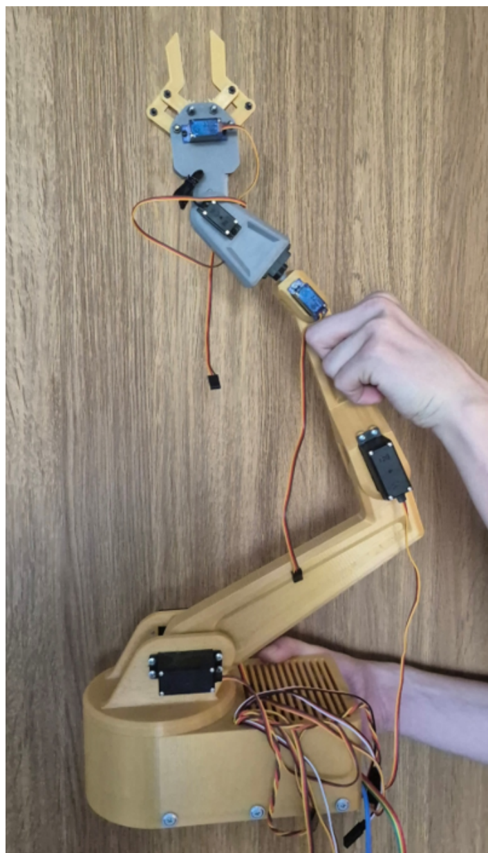
Obr. 6: Kompletná konštrukcia modifikovaného ramena
