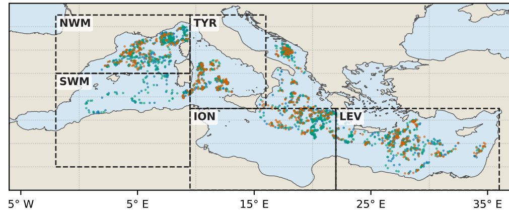
Test
