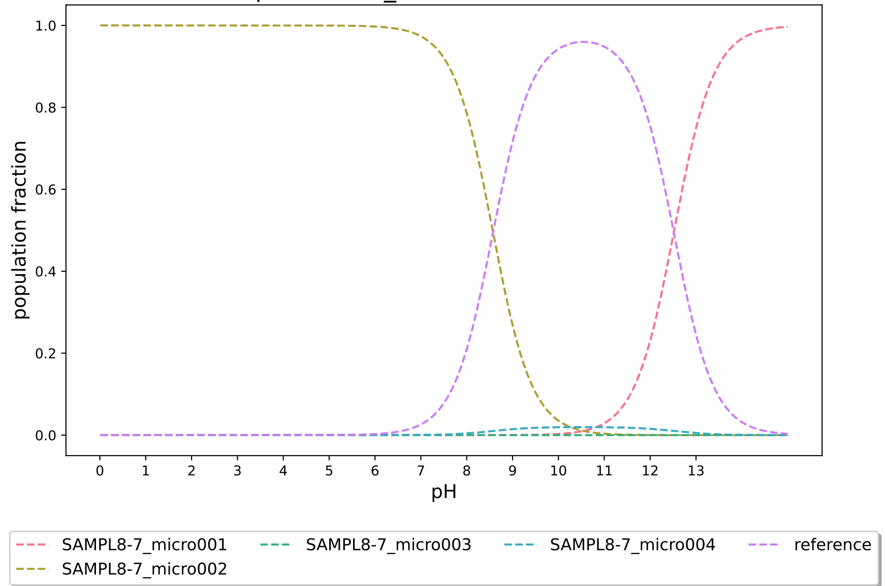
pKa-3DS-3_modified:SAMPL8-7
