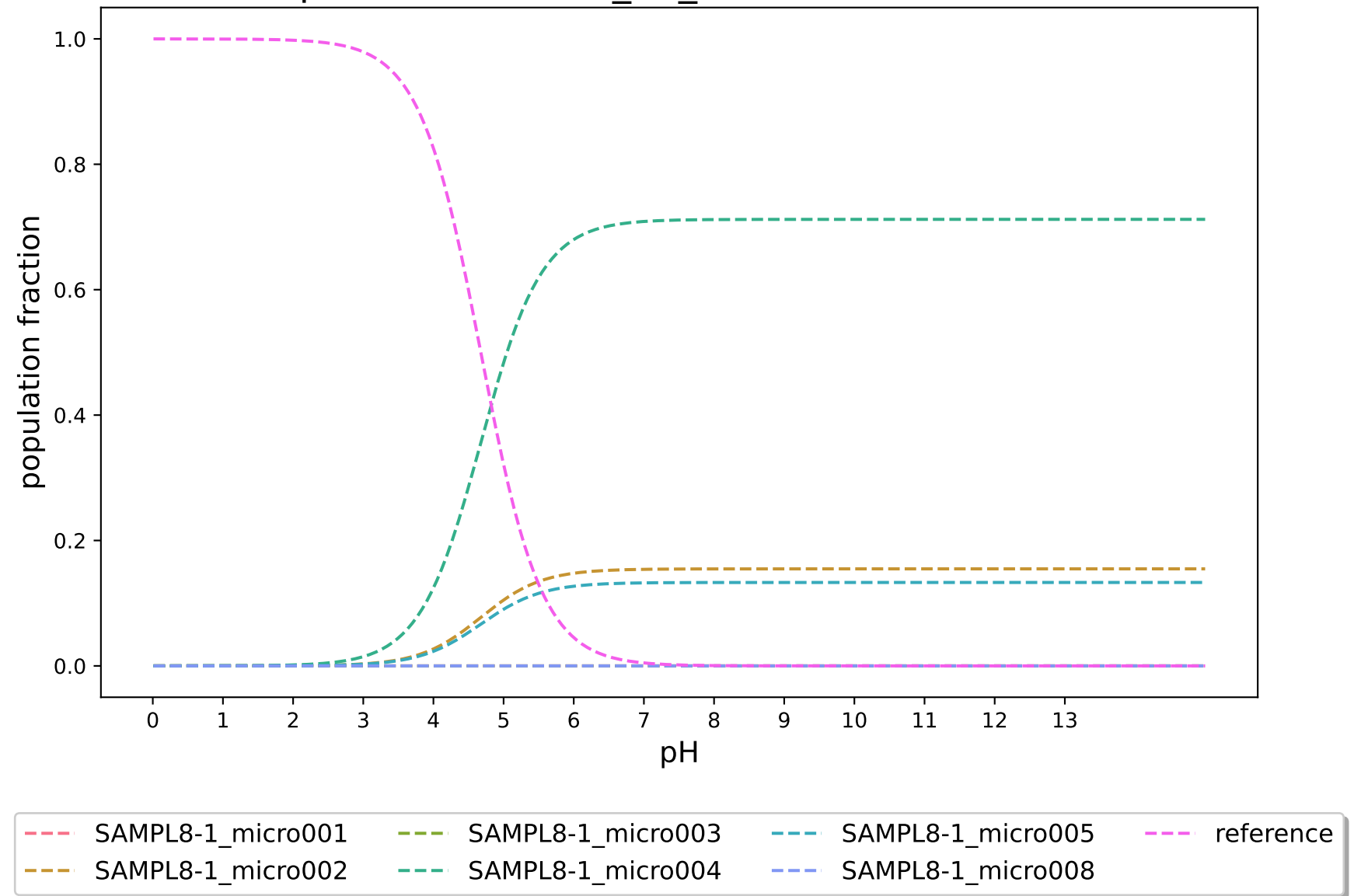
pKa-RobertRaddi_RF_modified:SAMPL8-1
