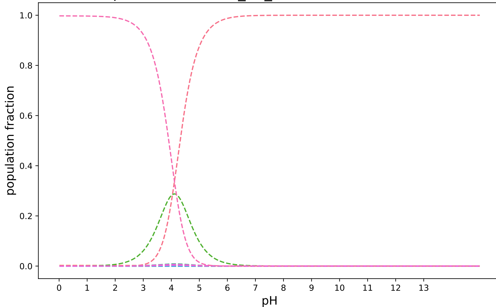
pKa-RobertRaddi_RF_modified:SAMPL8-14
