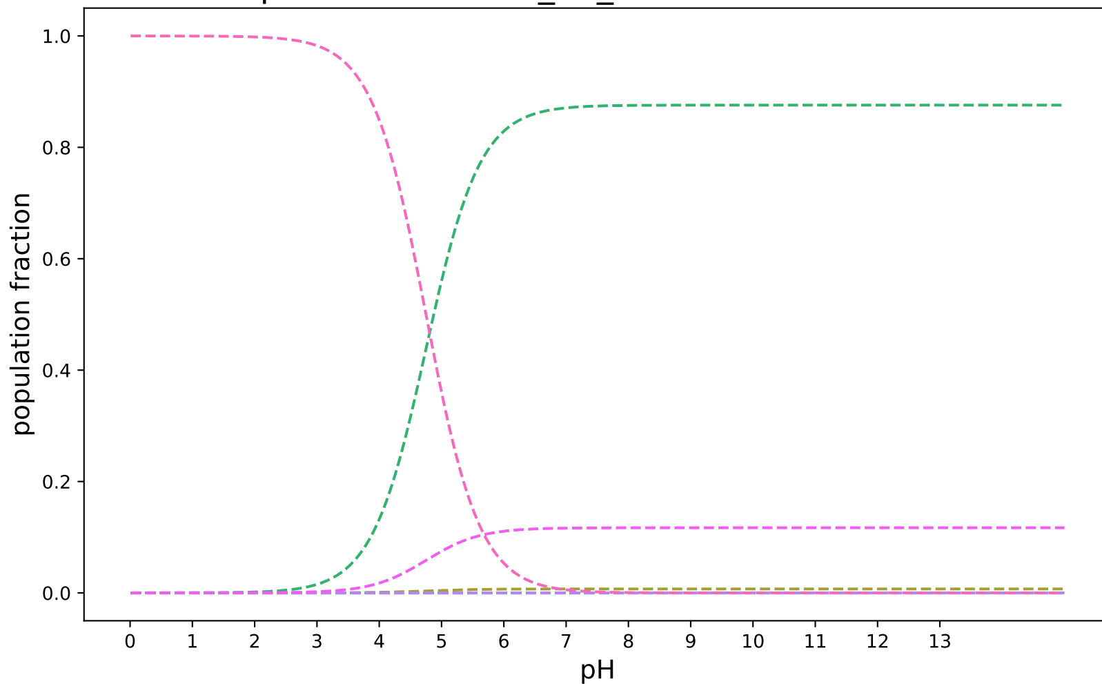
pKa-RobertRaddi_RF_modified:SAMPL8-3
