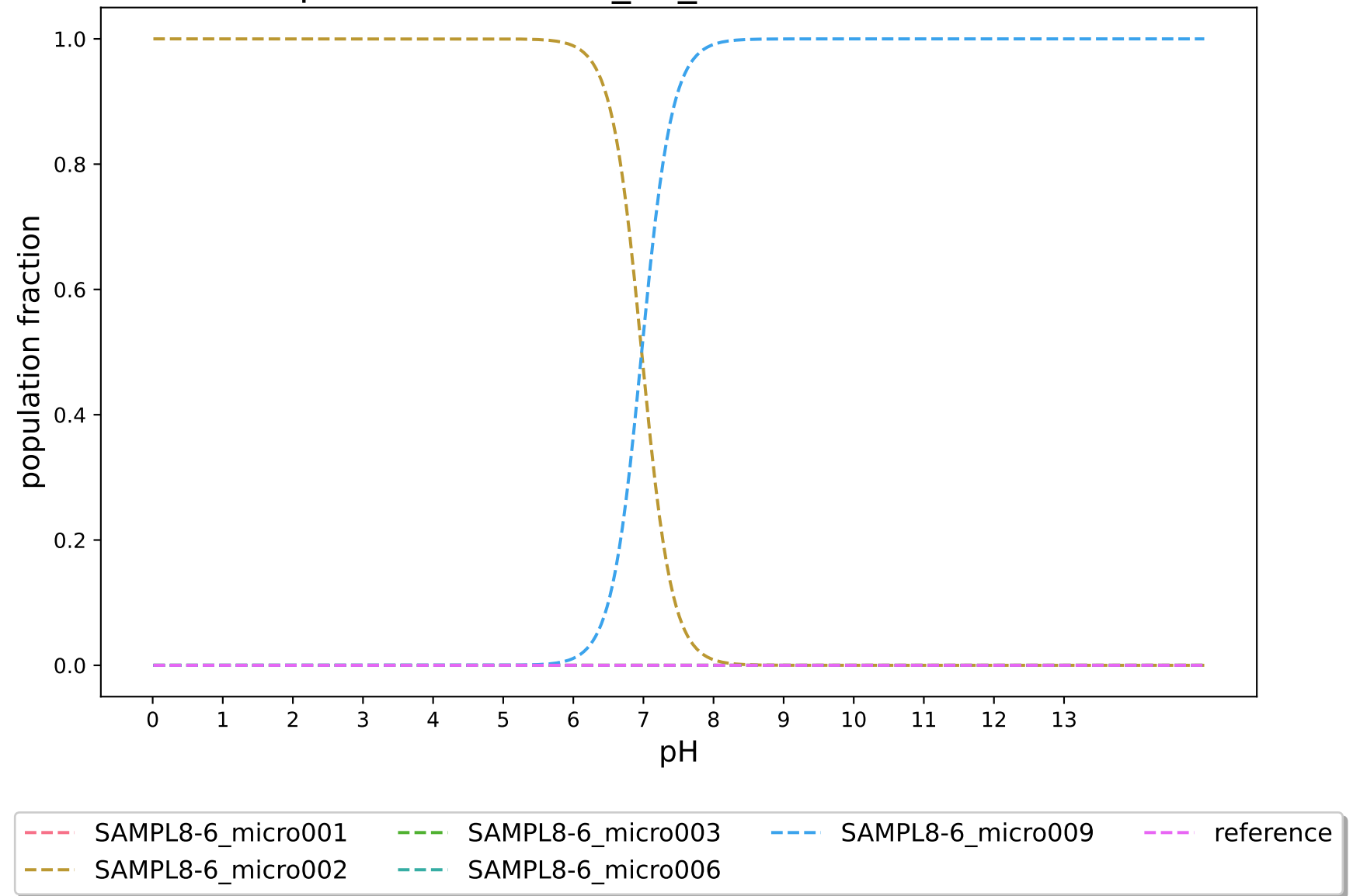
pKa-RobertRaddi_RF_modified:SAMPL8-6
