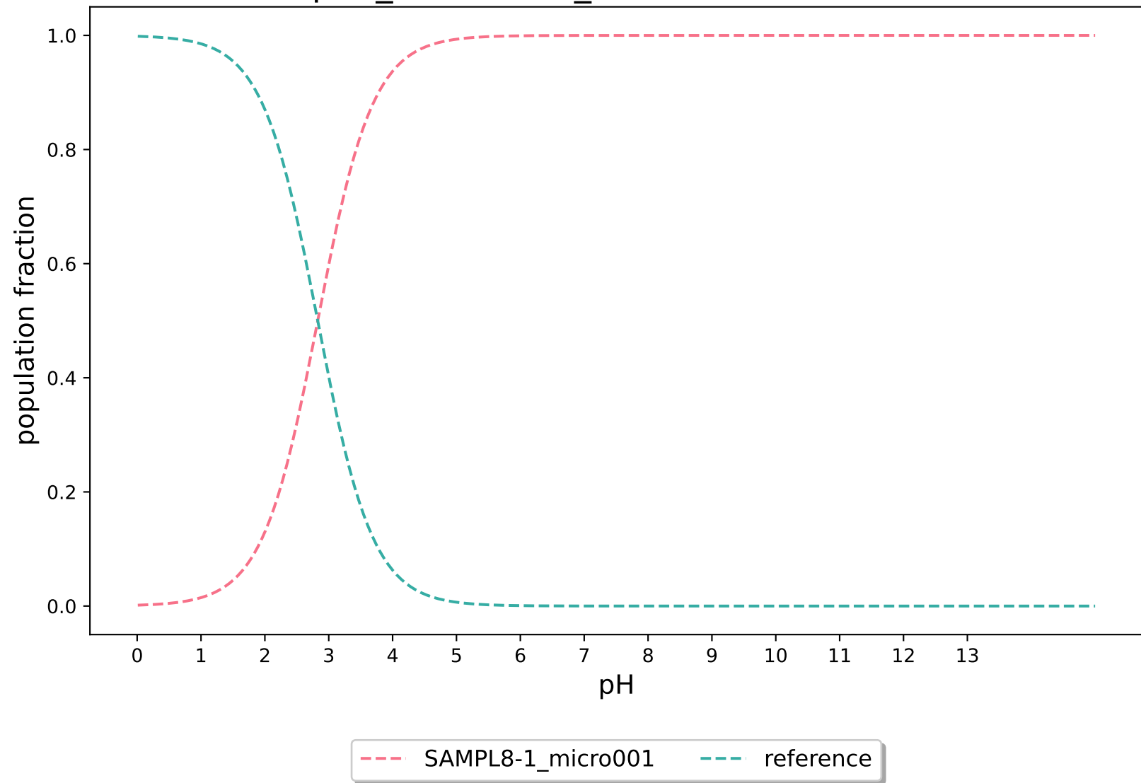
pKa_Chemaxon_modified:SAMPL8-1
