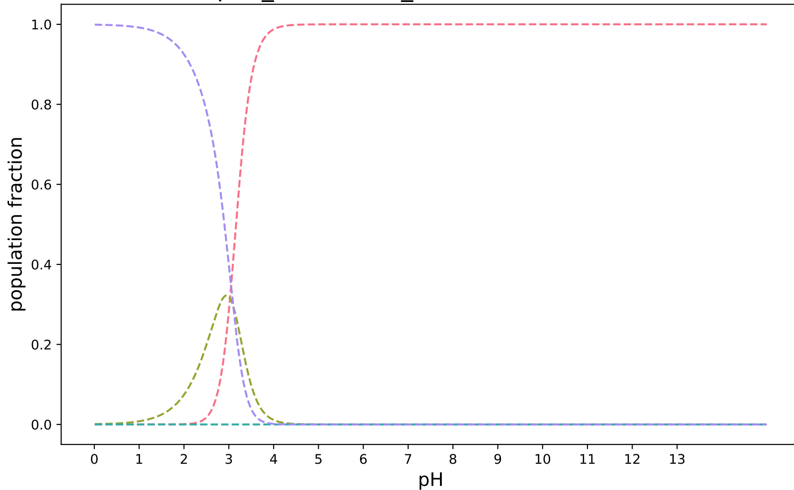
pKa_Chemaxon_modified:SAMPL8-3
