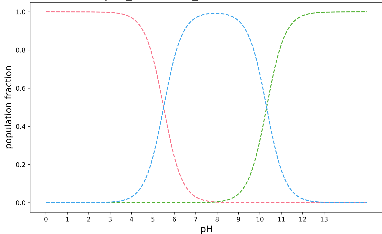
pKa_Chemaxon_modified:SAMPL8-7
