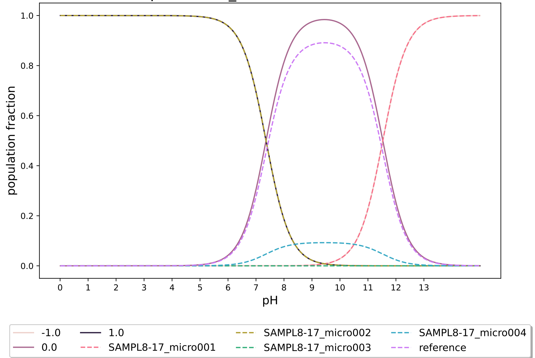
pKa-3DS-1_modified:SAMPL8-17
