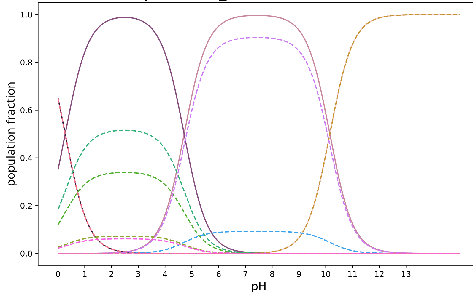
pKa-3DS-1_modified:SAMPL8-20
