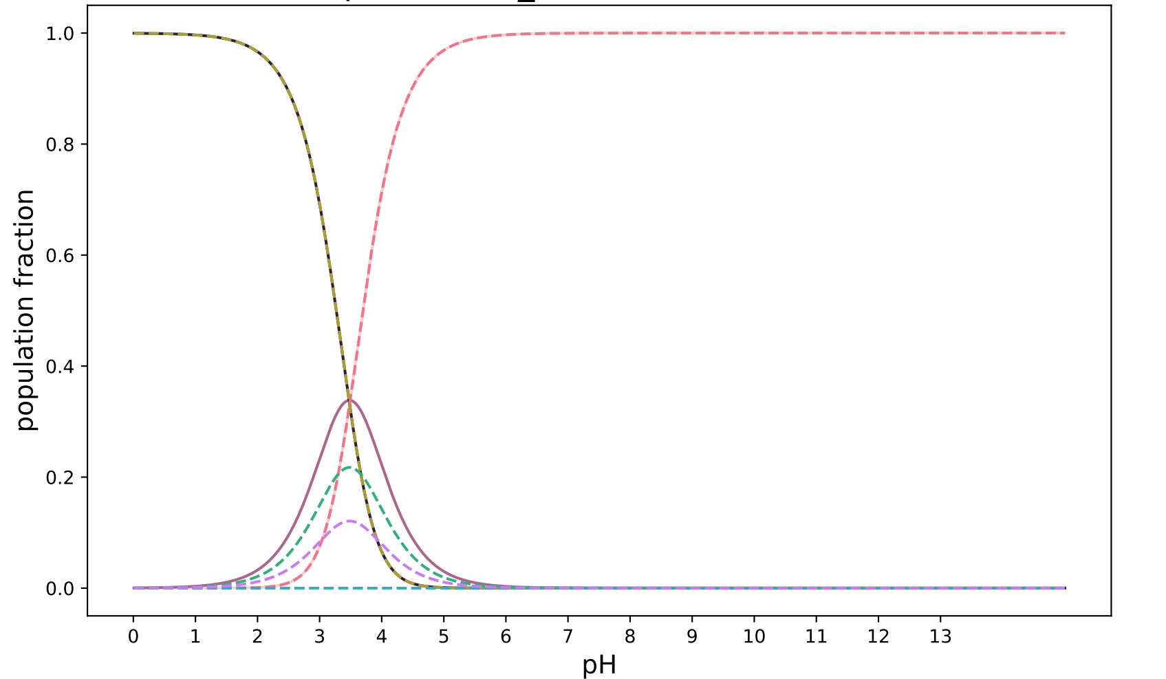
pKa-3DS-1_modified:SAMPL8-6
