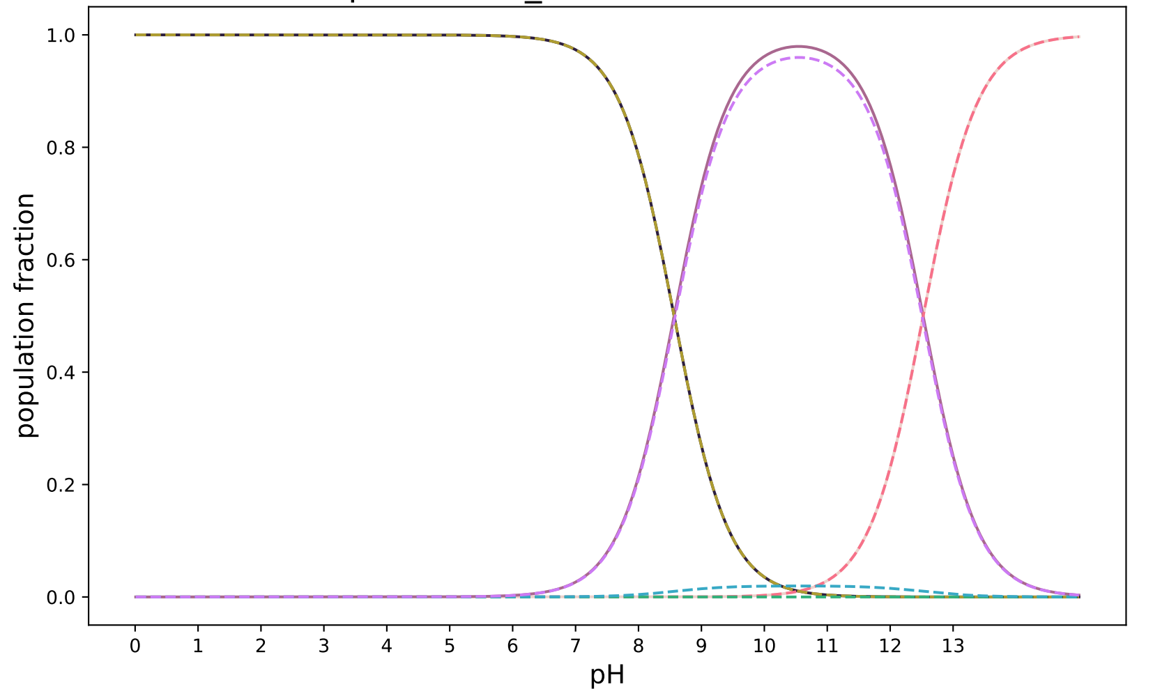
pKa-3DS-3_modified:SAMPL8-7
