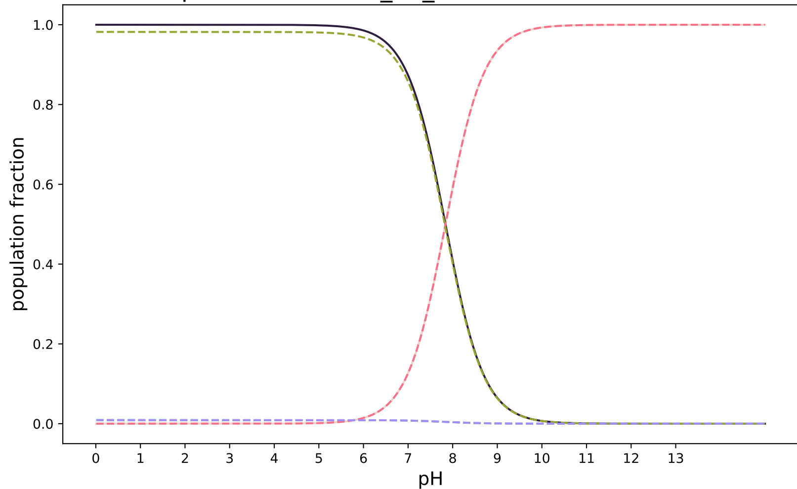
pKa-RobertRaddi_RF_modified:SAMPL8-22
