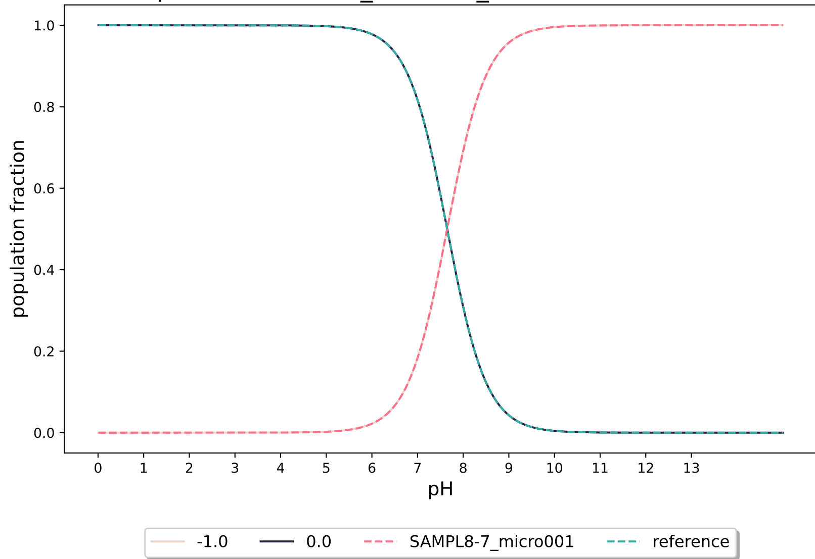
pKa-RobertRaddi_XGBoost_modified:SAMPL8-7
