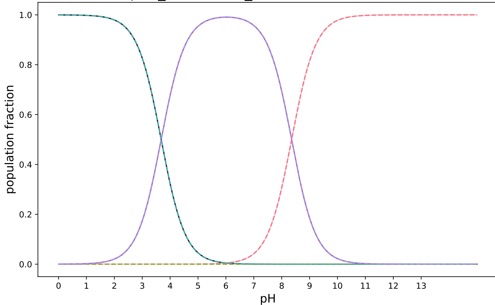
pKa_Chemaxon_modified:SAMPL8-16
