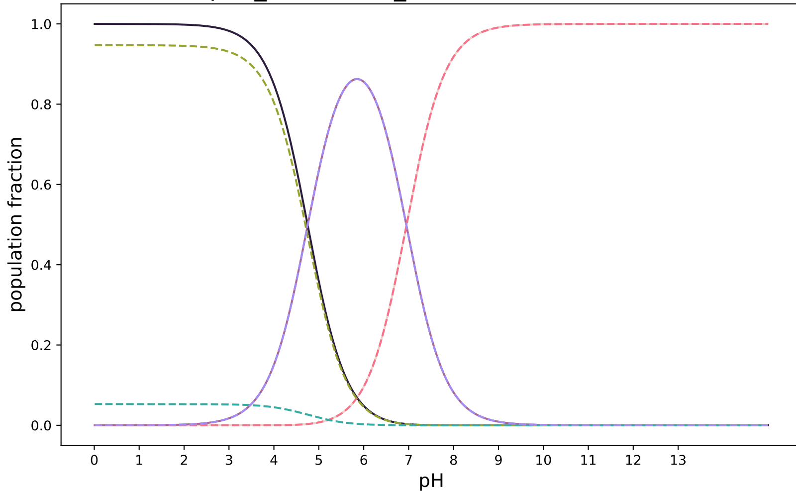
pKa_Chemaxon_modified:SAMPL8-19
